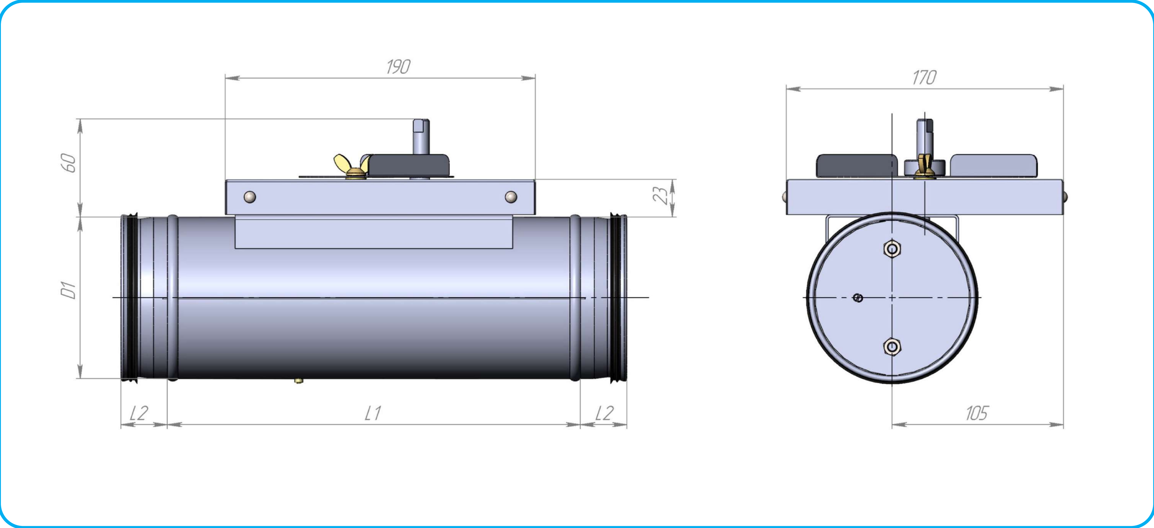
Рисунок 2. Типоразмеры клапана постоянного расхода воздуха КРК
