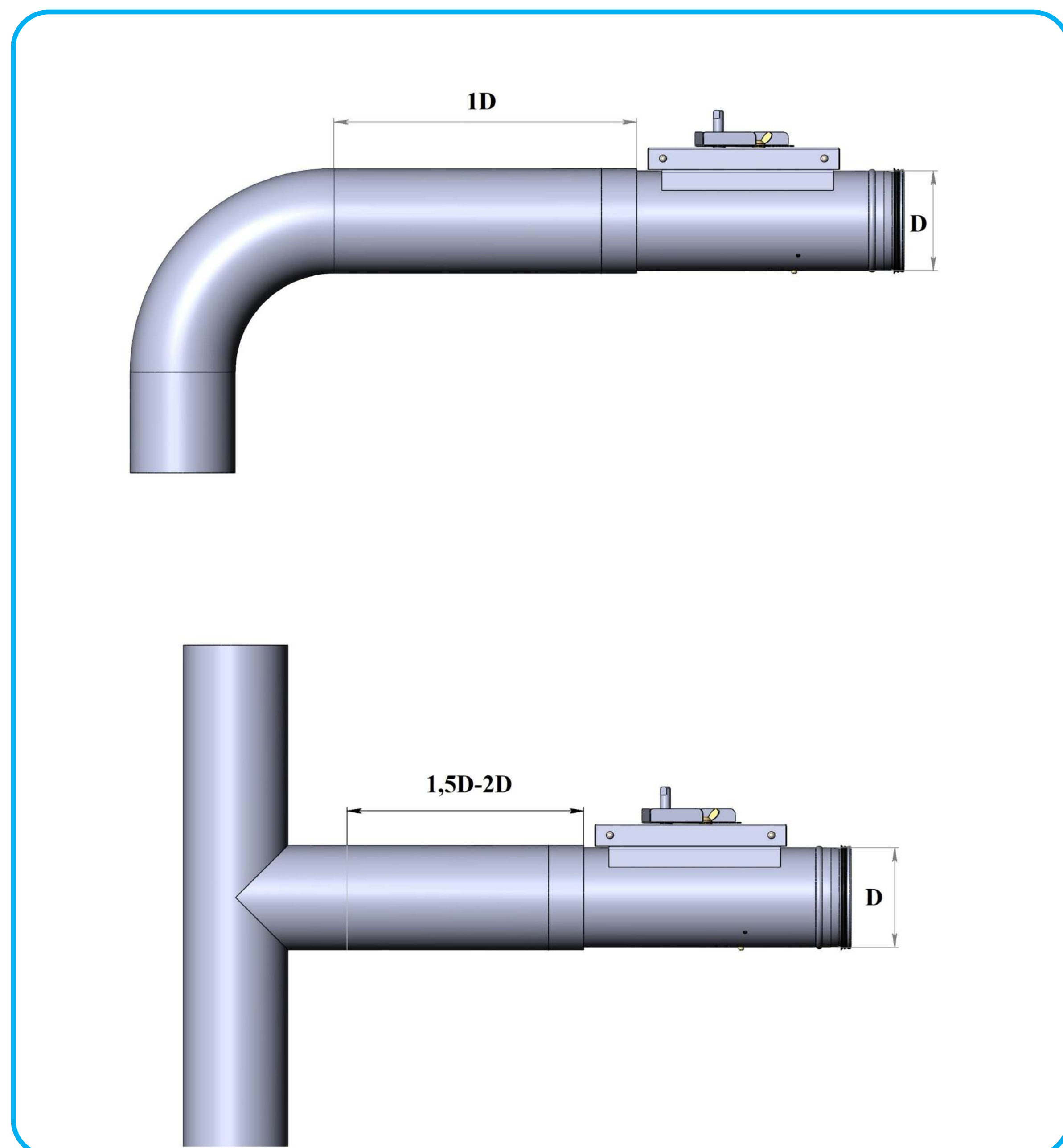
Рисунок 5. Настройка клапана
