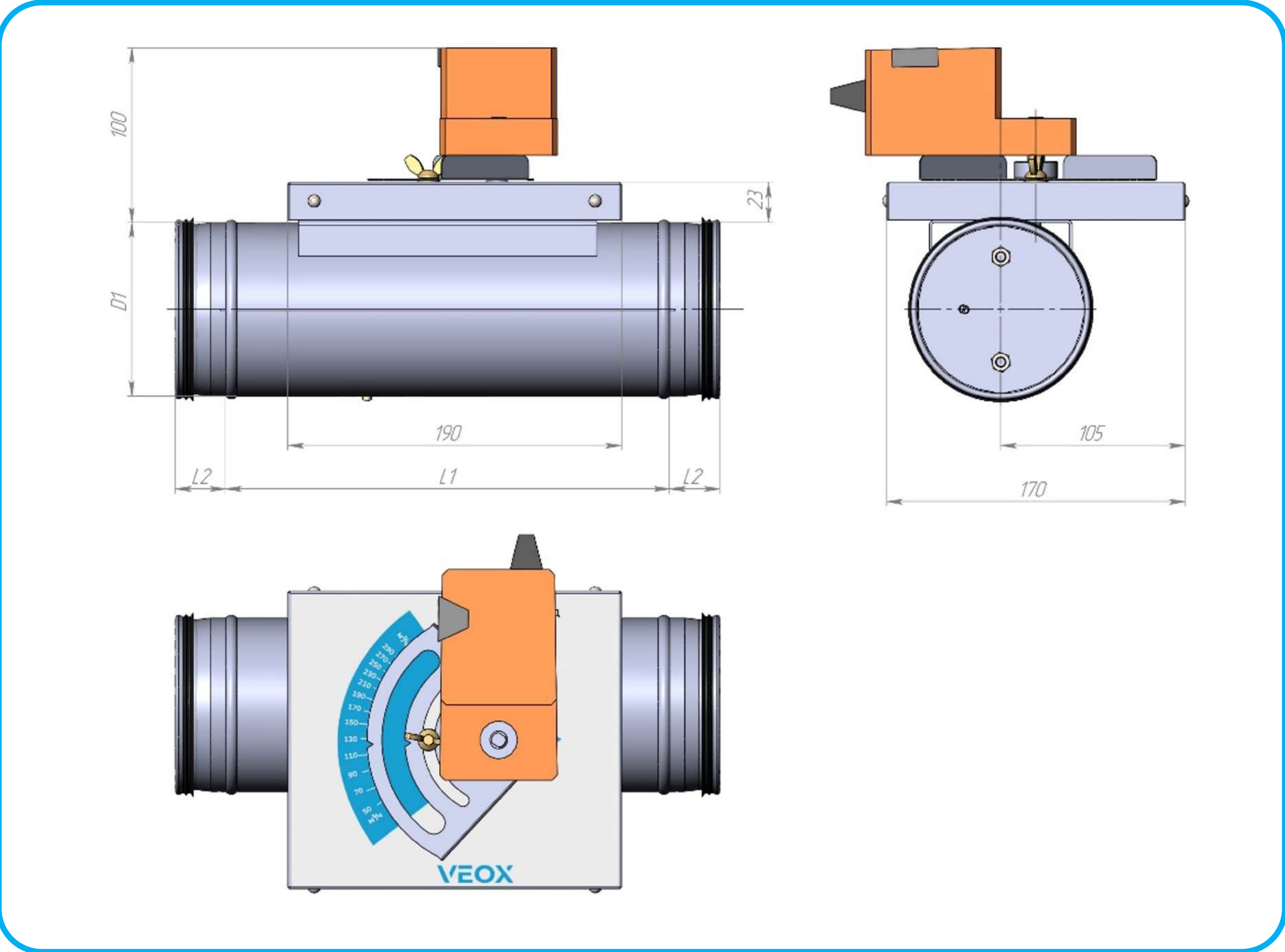
Рисунок 6. Вариант установки электропривода на клапан КРК
