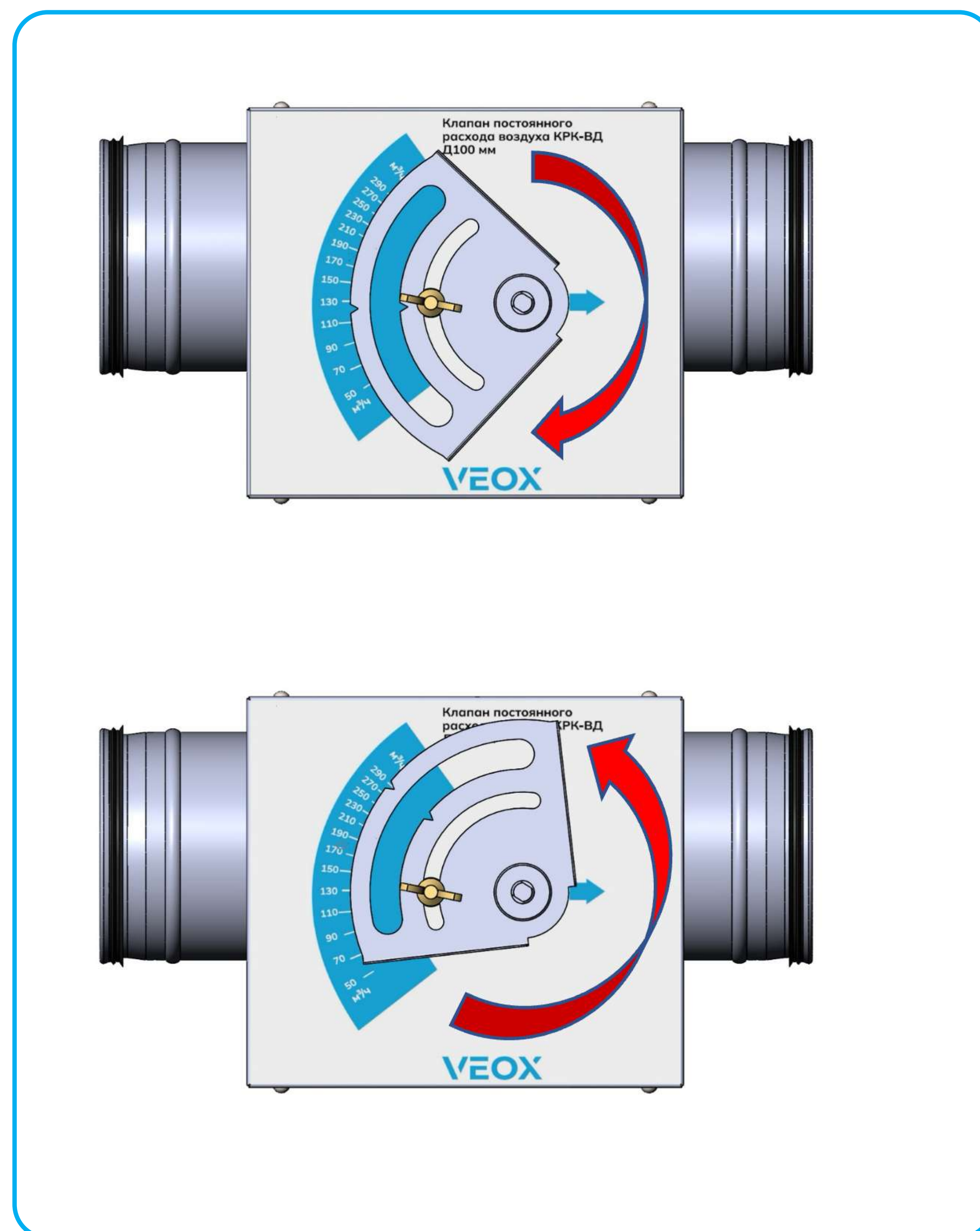
Рисунок 3. Настройка клапана
