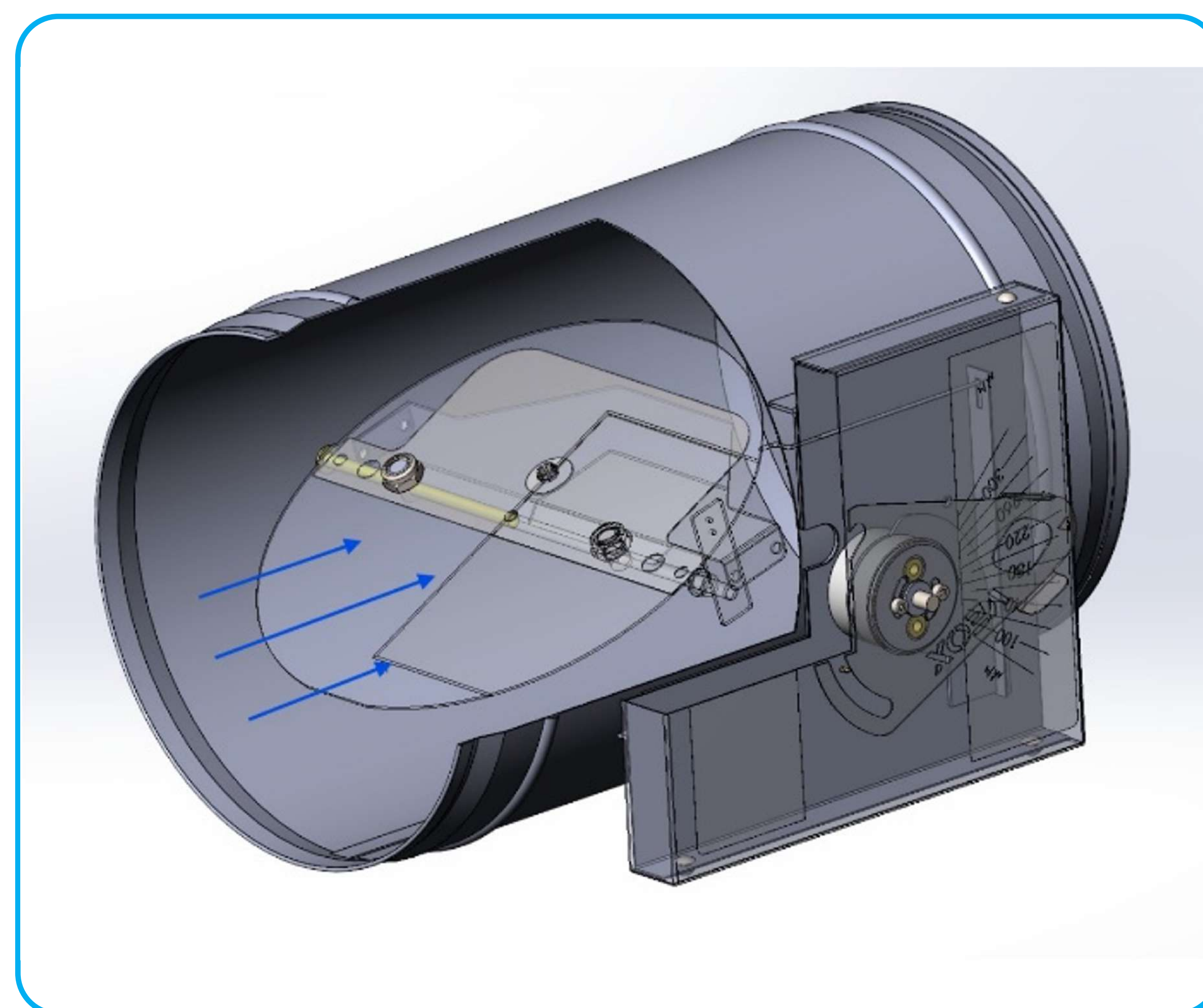
Рисунок 4. Конструкция клапана
